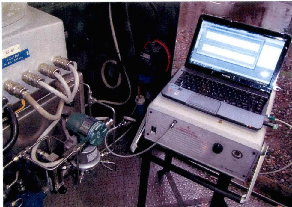
Foto 2 - Gascromatografo \mu GC 3000
