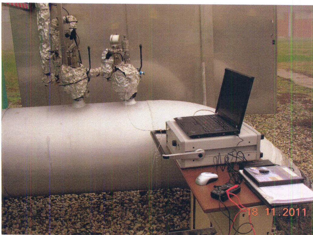
Foto 2 – Gascromatografo portatile µGC 3000 Agilent
