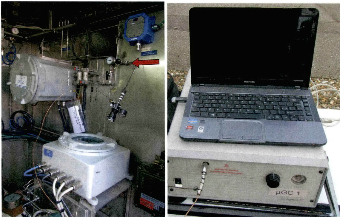
Foto 1 - Punto di campionamento (freccia di colore rosso) e gascromatografo portatile \mu GC 3000
