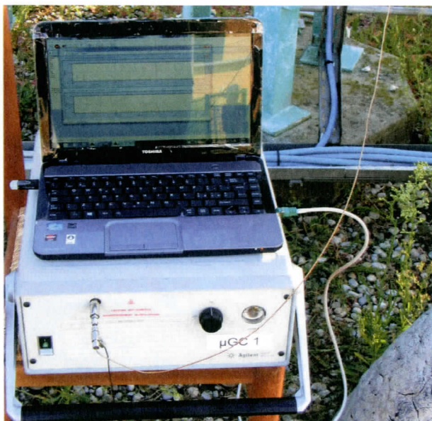
Foto 1 - gascromatografo portatile \mu GC 3000
