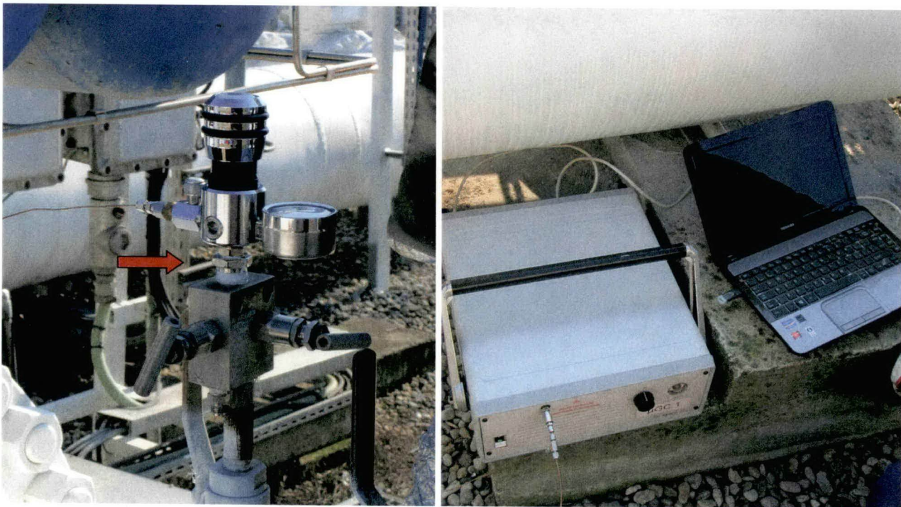
Foto 1 - Punto di campionamento (freccia di colore rosso) e gascromatografo portatile \mu GC 3000
