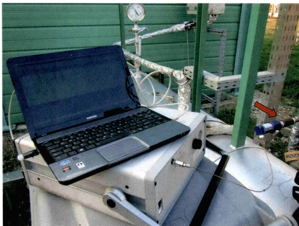
Foto 1 - Punto di campionamento (freccia di colore rosso) e gascromatografo portatile \mu GC 3000
